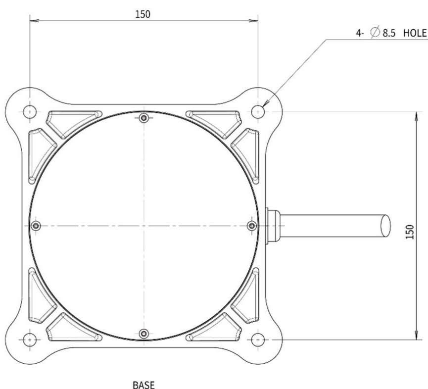
Dessin de la base du manipulator, utiliser quatre boulons M8. Unité [mm]
